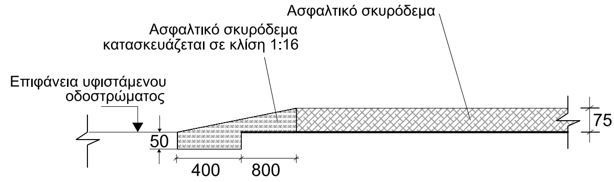
ΤΟΜΗ Α-Α διαστάσεις σε χιλιοστά
