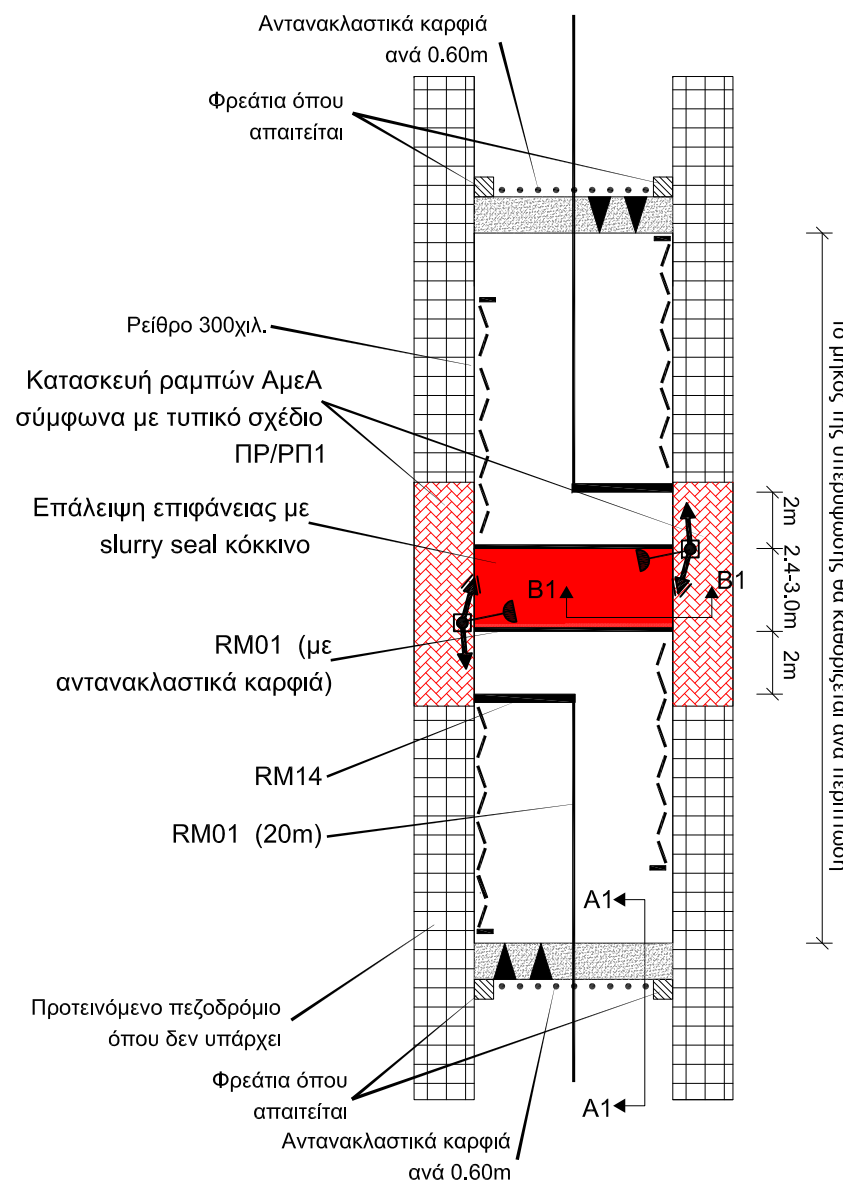
ΚΑΤΟΨΗ ΦΩΤΟΕΛΕΓΧΟΜΕΝΗ ΔΙΑΒΑΣΗ ΠΕΖΩΝ PELICAN ΣΕ ΥΠΕΡΥΨΩΜΕΝΟ ΠΛΑΤΟ ΑΠΟ ΑΣΦΑΛΤΙΚΟ
